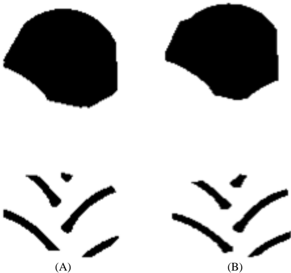
Figura 3. Área de contato e de garras radial (A), área de contato e garras radial IF (B),
